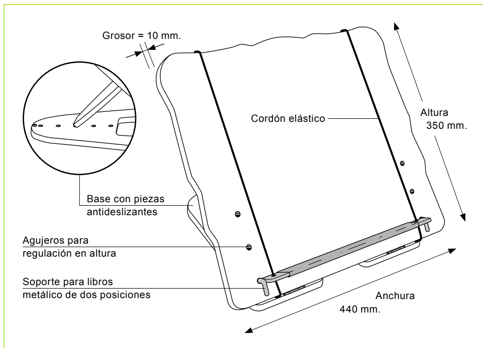
Esquema técnico
