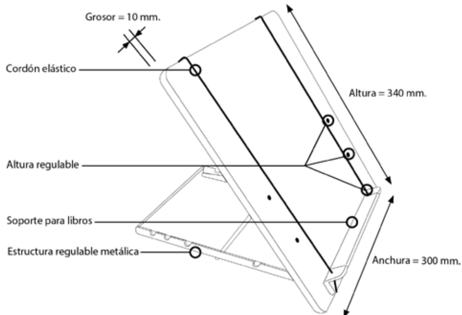
Esquema técnico
