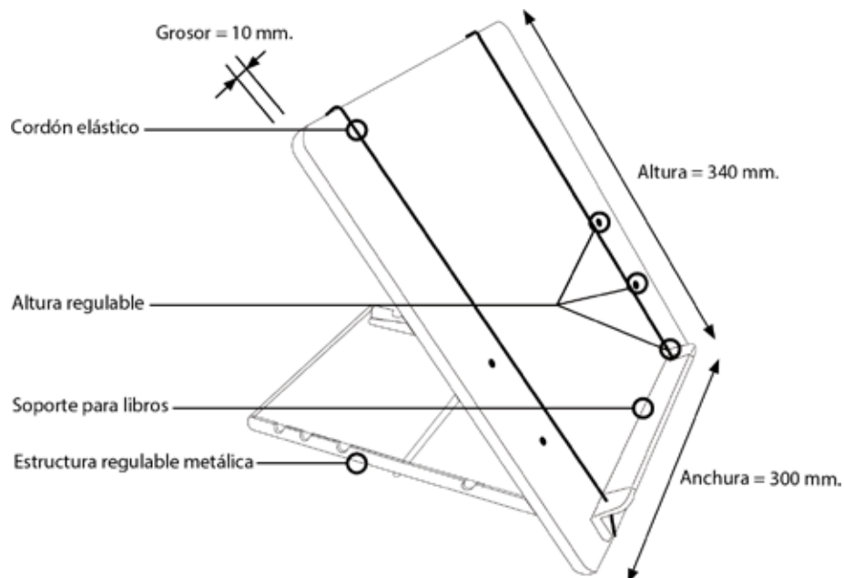
Esquema técnico
